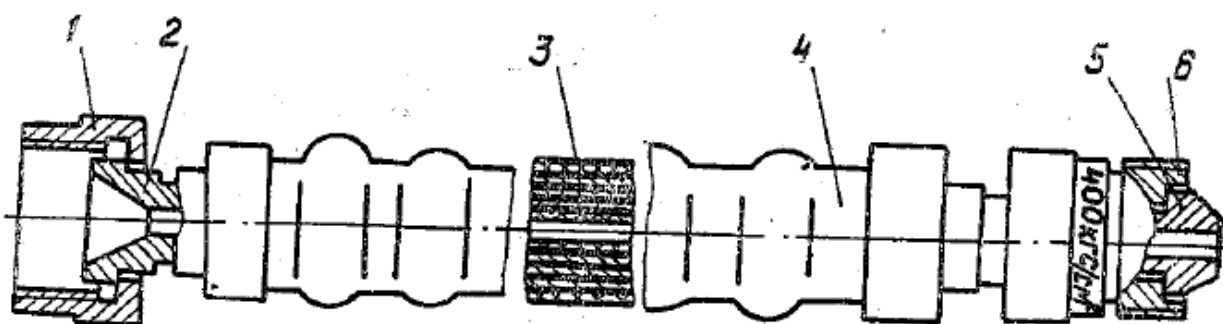
Рис. 21. Шланг высокого давления Сб 0701:
