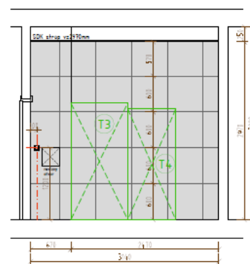
REZOPOHĽAD J
