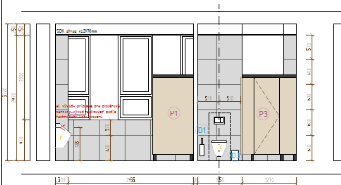
REZOPOHĽAD G
