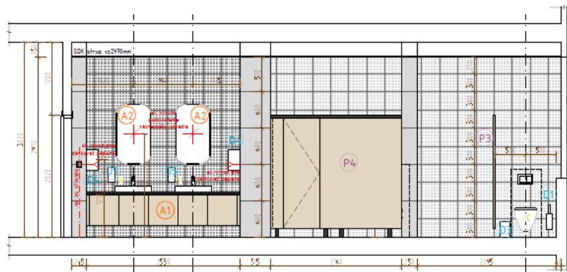
REZOPHĽAD D – s deliacimi priečkami
