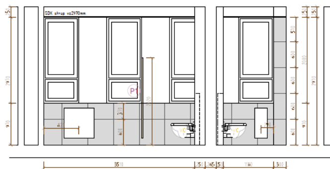
REZOPHĽAD E
