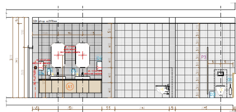
REZOPHĽAD D – bez deliacich priečok
