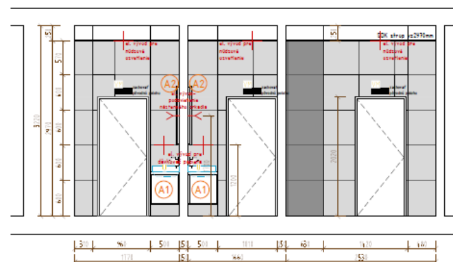
REZOPOHĽAD H
