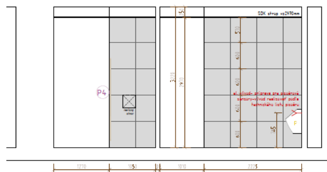
REZOPHĽAD F
