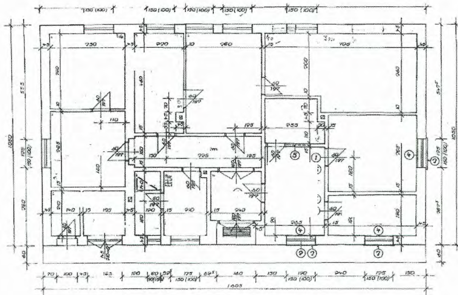
BUDOVA ČÍSLO 33 SÚP. Č. 300 NA PARC. Č. 288/13 - PÔDORYS
