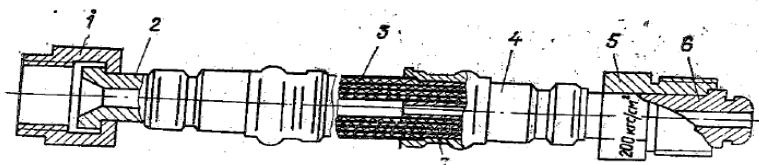
Рис. 22. Шланг Сб 0702В/5Л191:
