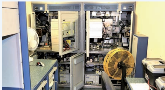
Pohľad do kontajnerov s výpočtovým a prístrojovým vybavením nového a starého približovacieho rádiolokátora
