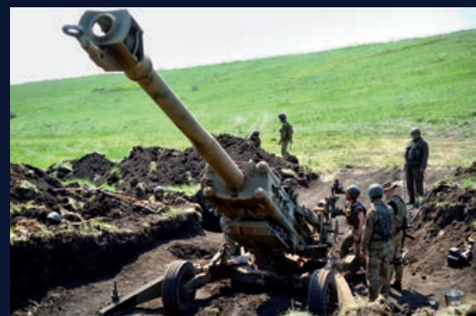
Ťahaná ľahká poľná húfnica 155 mm M777
