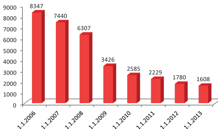
Graf č. 2: Vývoj počtu profesionálnych vojakov ozbrojených síl, ktorých vojenská služba trvá menej ako 5 rokov.
