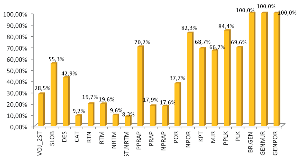
Graf č. 3: Percentuálny počet profesionálnych vojakov po jednotlivých hodnotiach, ktorí boli ku dňu 31. 12. 2013 na platovom strope.
